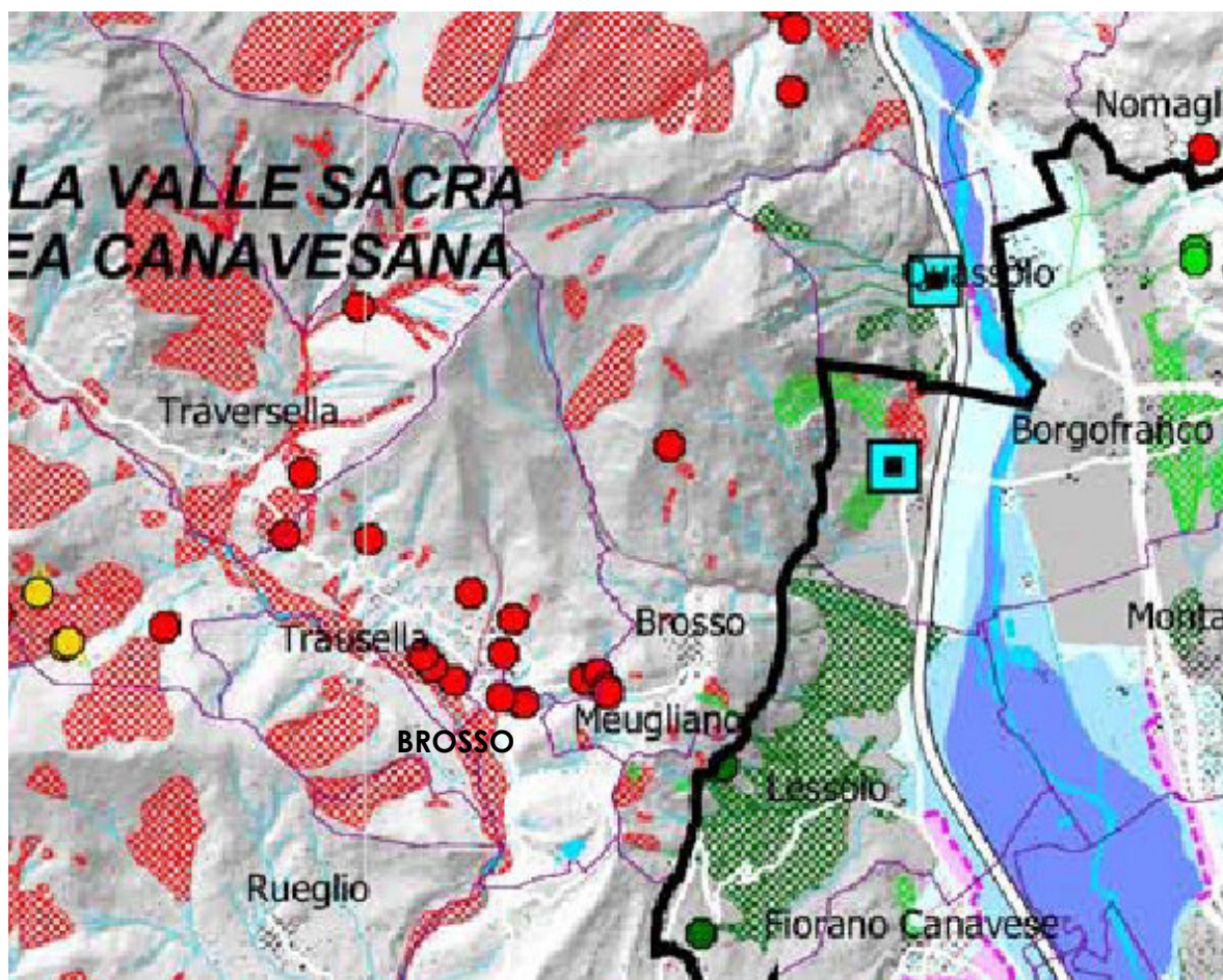
Estratto della Tavola 5.1 del PTC2 "Dissesto idrogeologico, comuni sismici e abitati da trasferire e consolidare."
