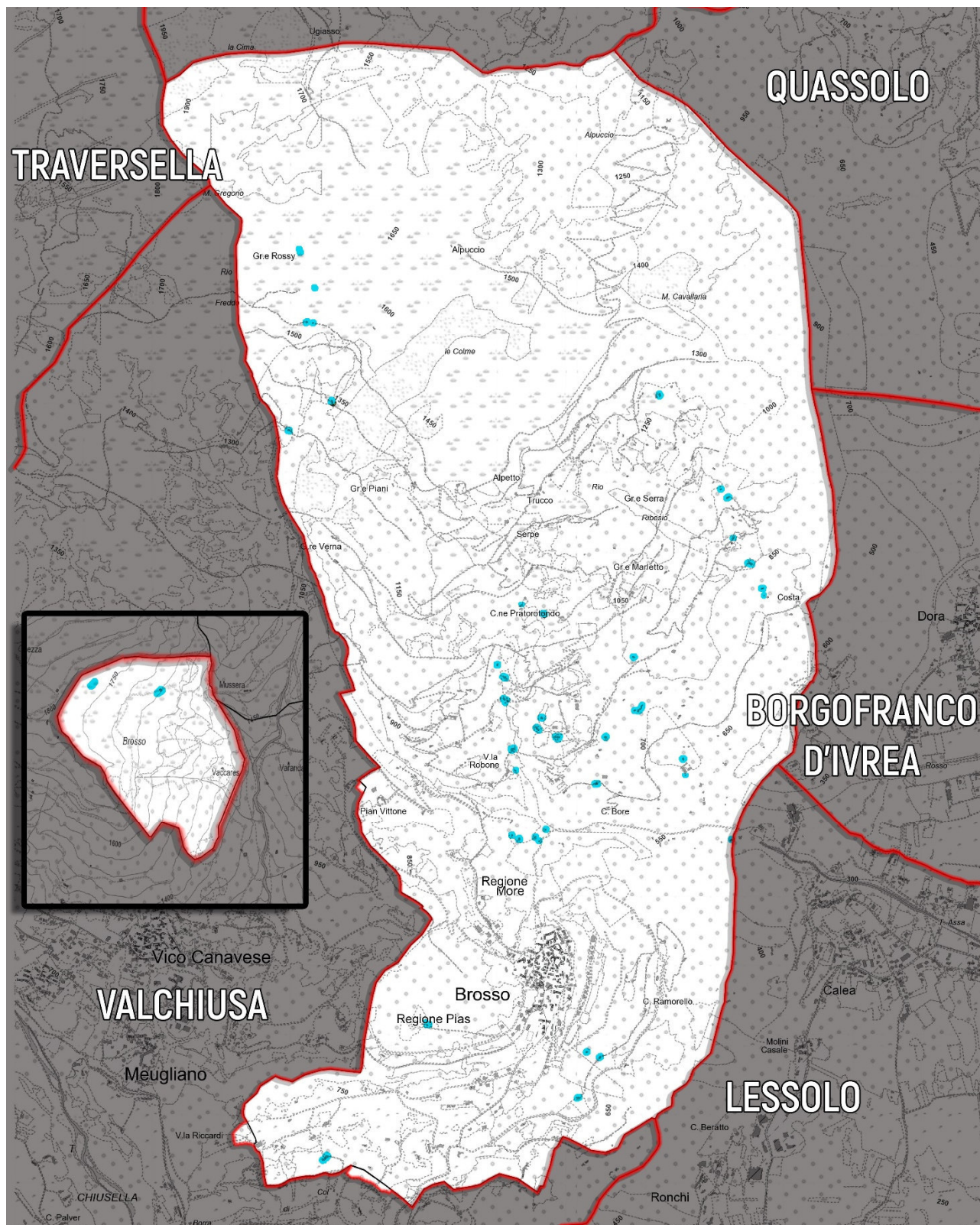
Carta Tecnica Regionale del Comune di Brosso con evidenziata la classe IIIb4 di pericolosità geomorfologica.
