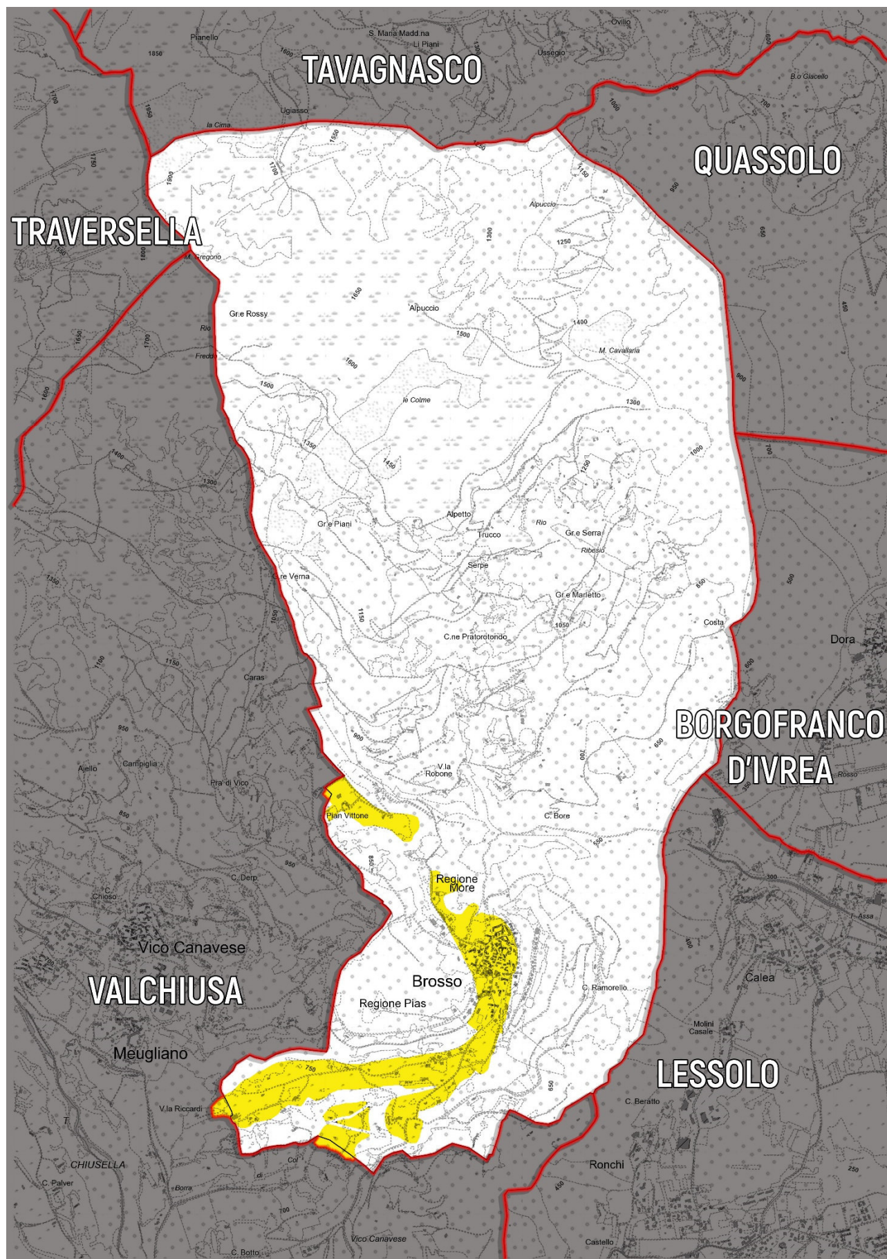
Estratto della BD3 del territorio comunale di Brosso, con evidenziata la classe IIa di pericolosità geomorfologica.
