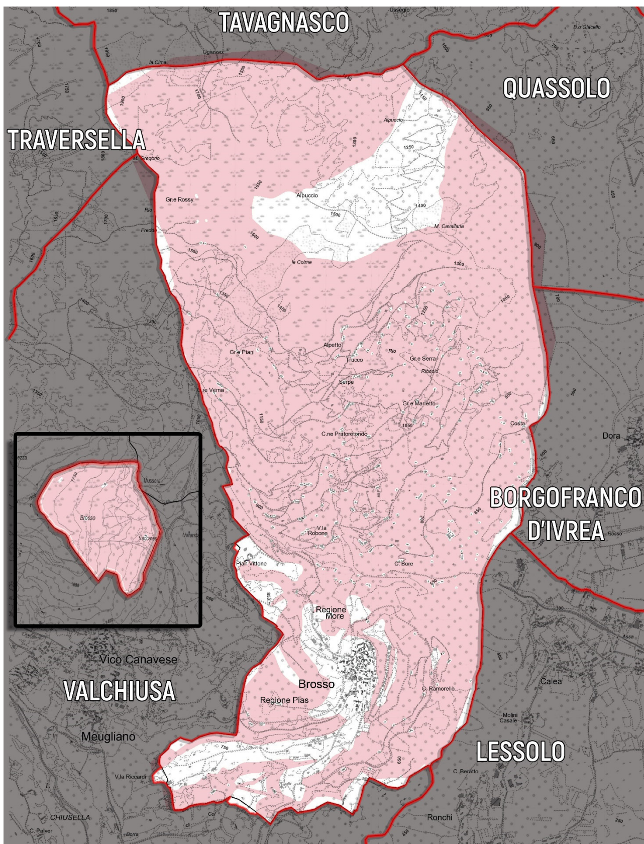
Estratto della BD3 del territorio comunale di Brosso, con evidenziata la classe IIIa di pericolosità geomorfologica.
